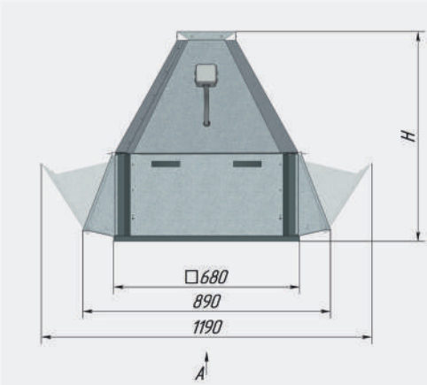
Габаритные и присоединительные размеры
